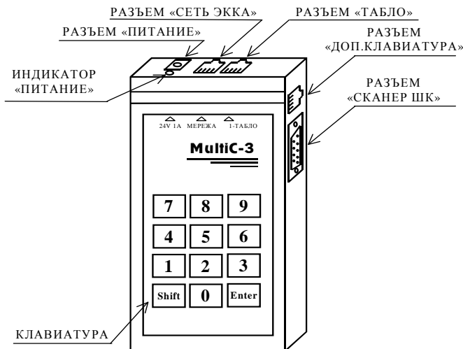
Рисунок 1 Контроллер «MultiC-3.1»
