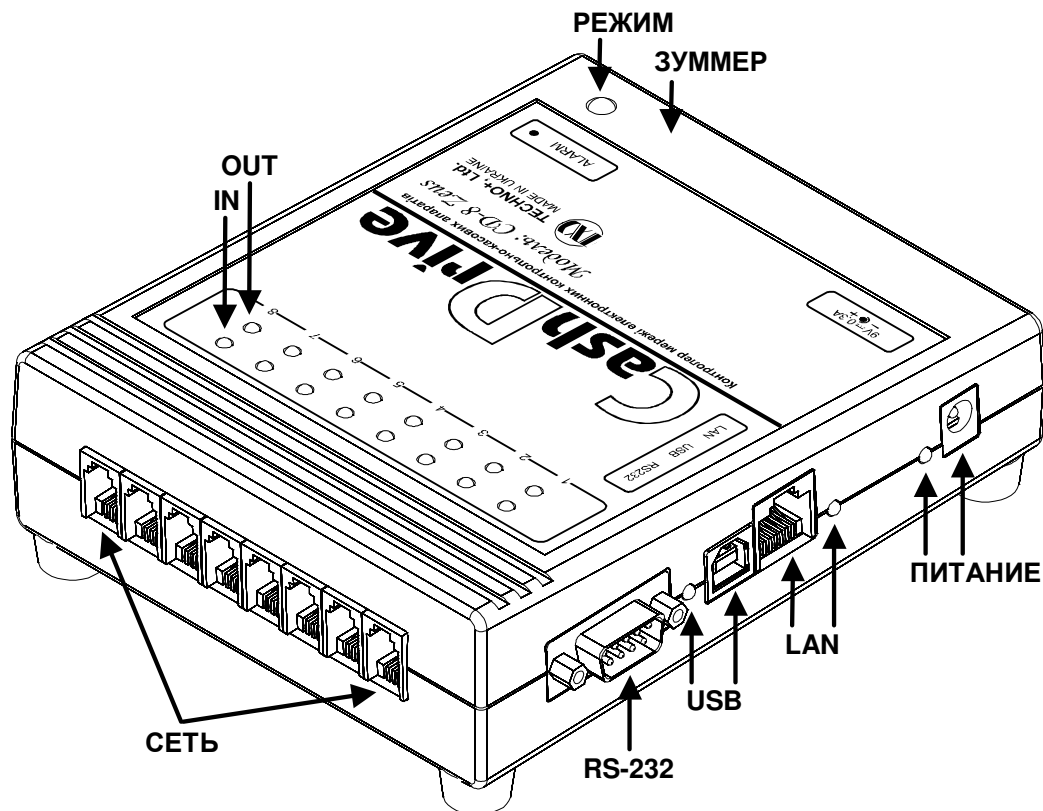
Рисунок 1 Контроллер «CashDrive CD-8 Zeus»
